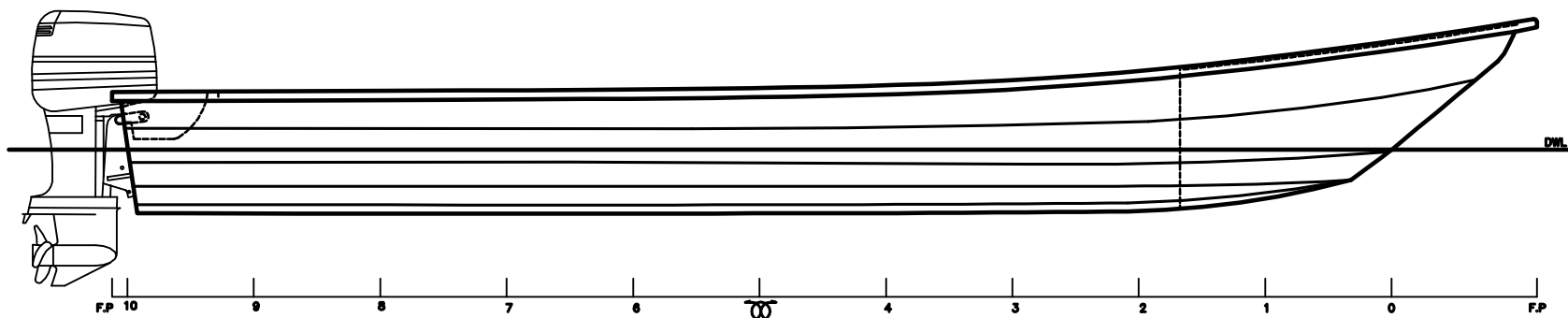
PERFIL EXTERIOR
